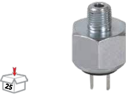
🇹🇷 08-023 Üniversal Hidrolik Fren Müşürü M10X1 (3,5 bar)
